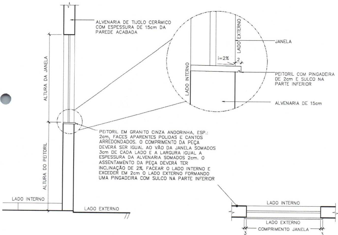
DETALHE 4 ESCALA 1:20 TÍPICO PINGADEIRA
