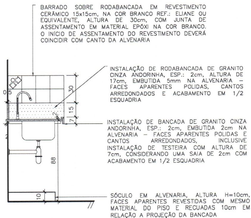
DETALHE 1 ESCALA 1:20 TÍPICO BANCADA MOLHADA
